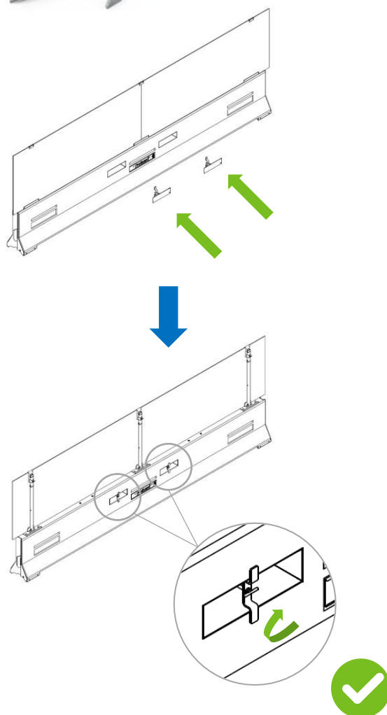
Lock Gaffelficka Art.no 10280
